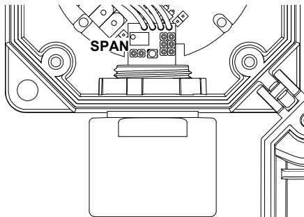
Fig. 9b: Posición del control de Span en el sensor para gases Tóxicos.
