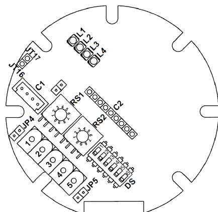
Fig. 5: Disposizione interna.
